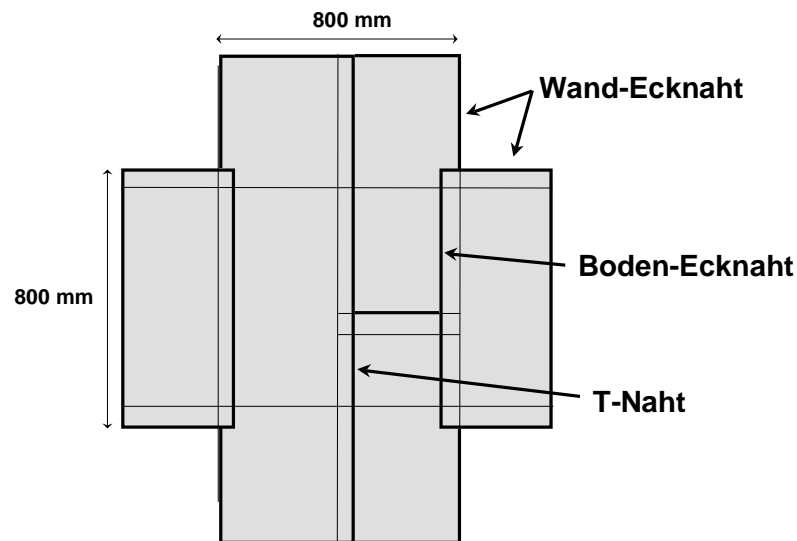
Abb. 1: Im FLL-Verfahren vorgesehene Ausführung der Nähte
