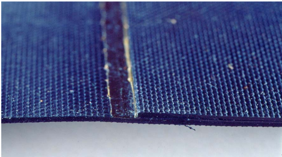
Abb. 4: Schnitt durch Längsnaht (Detail)
