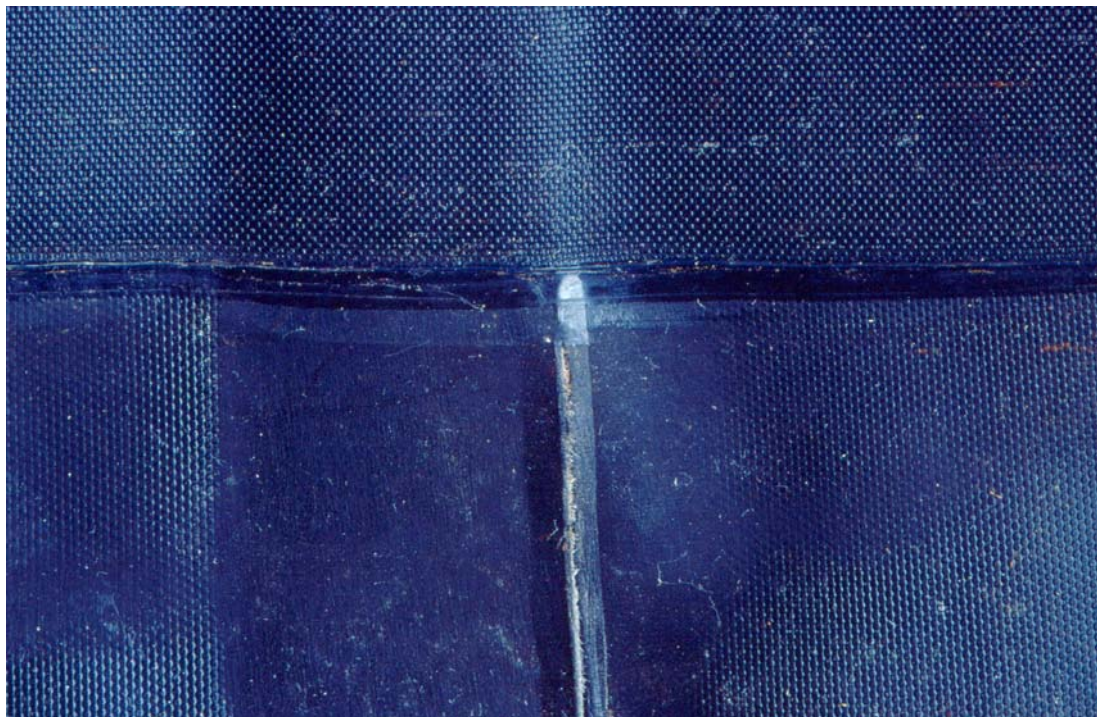
Abb. 2: Bahnoberseite mit T-Naht
