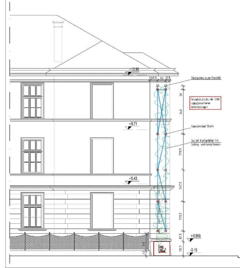
Teilansicht: Andreas Hofer-Straße M 1:100
