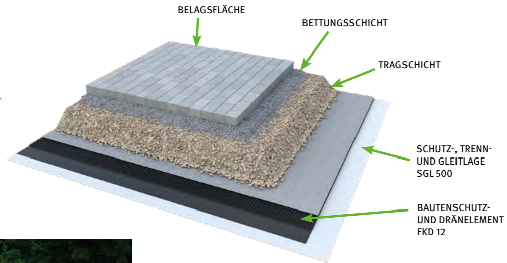
Beispielhafter Aufbau eines Verkehrsdachs Nutzungskategorie 2 - befahrbare Dachflächen für PKW
